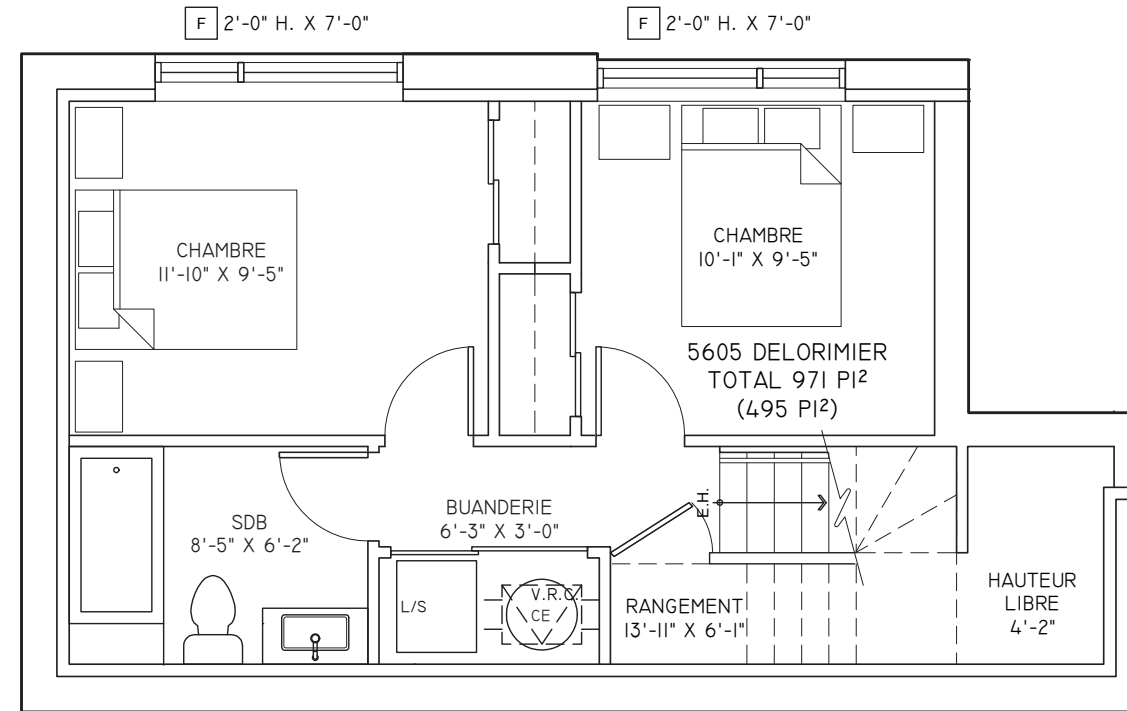
REZ-DE-JARDIN 495 PI 2
