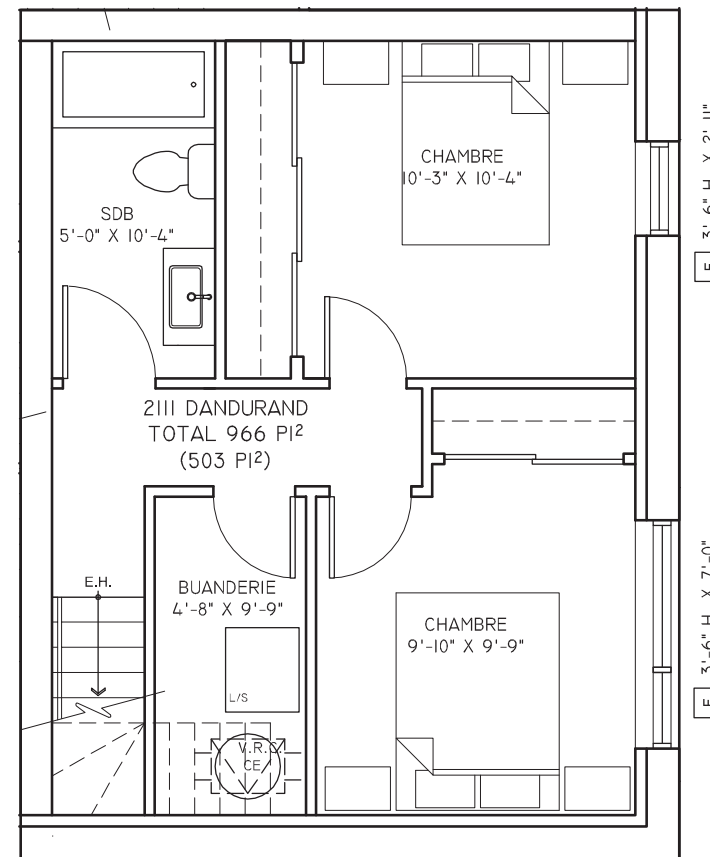
REZ-DE-JARDIN 503 PI 2
